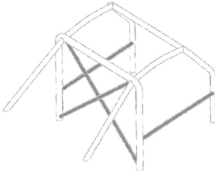
Obr. - Minimální konstrukce ochranného rámu
