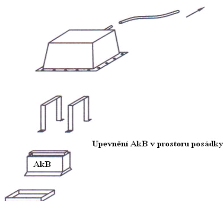
Obr.- Upevnění a zakrytování AkB v prostoru posádky
