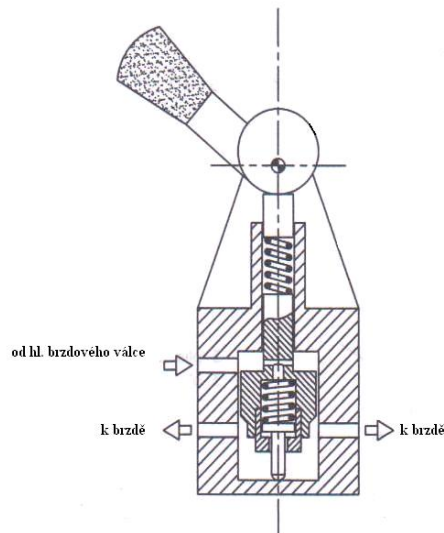
Obr. - Rozdělovač brzdného účinku
